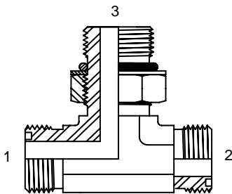
(1) (2) MALE ORFS (3) ADJ. O-RING
